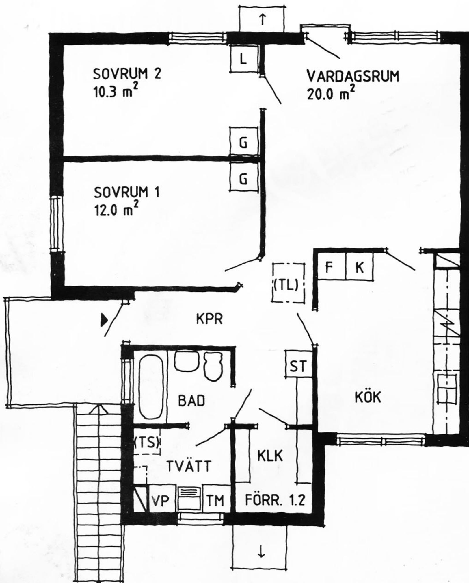
TYP 3B ÖVRE PLAN
