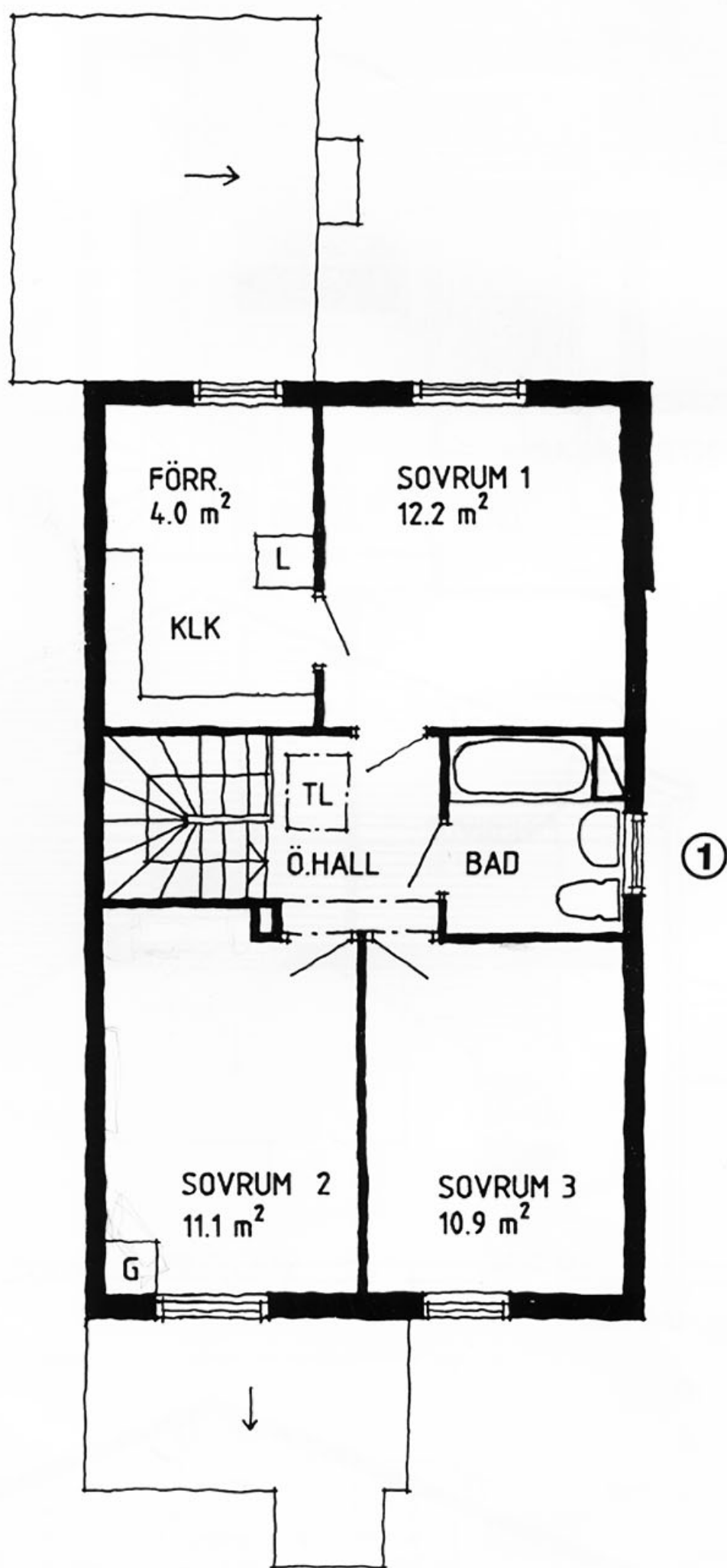
ÖVRE PLAN
